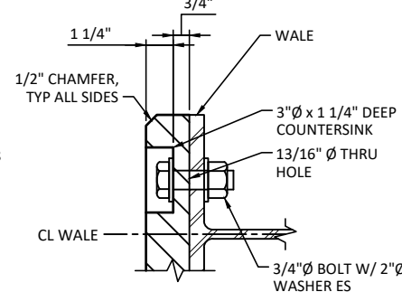
H SECTION - WALE RUB STRIP SCALE: 3" = 1'-0"
