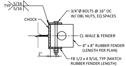
J SECTION - RUBBER FENDER SCALE: 1 1/2" = 1'-0"
