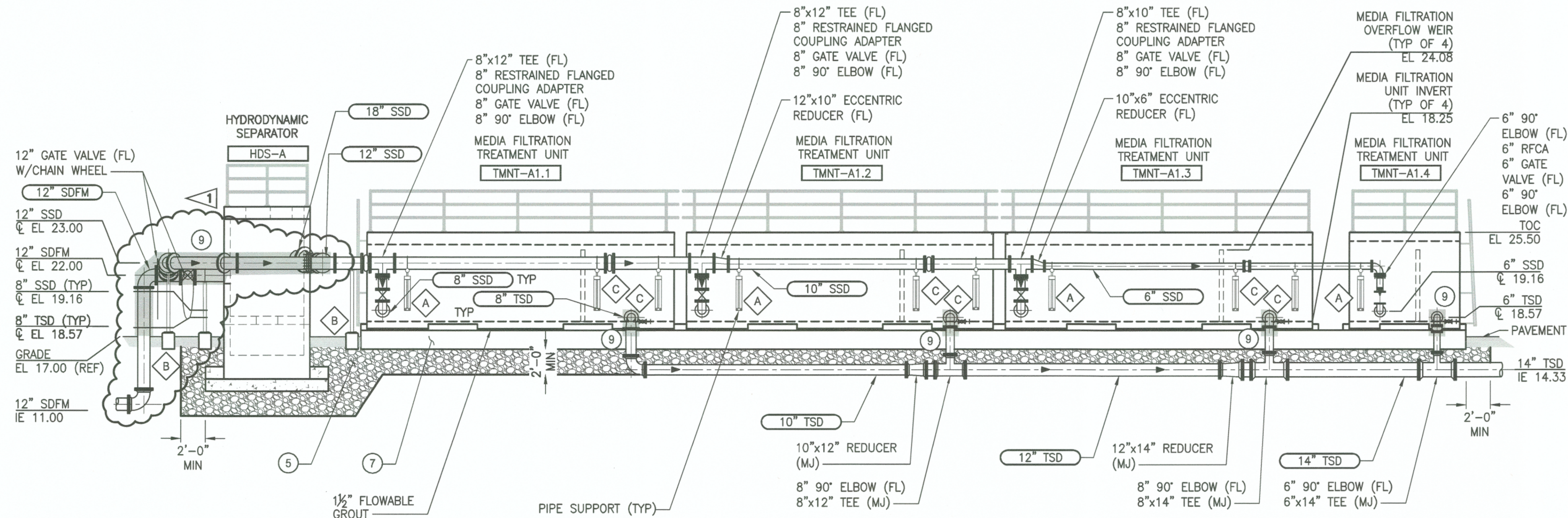
C SECTION SCALE: 3/16"=1'-0"
